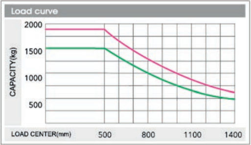
CPCD 15
